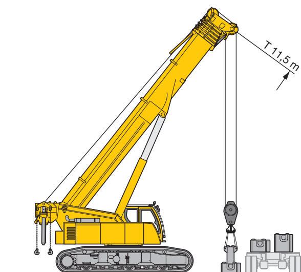
Montage Drehbühnenballast Assembly superstructure ballast Montage du contrepoids de la partie tournante Montaggio zavorra piattaforma girevole Montaje contrapeso superestructura Монтаж противовеса поворотной илатформы
